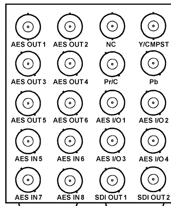
RM-9034-D
